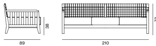
SYDI Sofa / Divano / Canapé / Sofa SYCUSE Cushion / Cuscino Coussin / Sitzpolster
