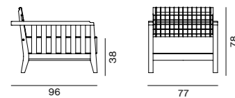
SYPO Armchair / Poltrona Fauteuil / Sessel SYCUSE Cushion / Cuscino / Coussin Sitzpolster
