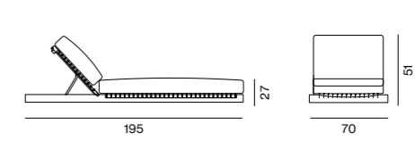
SYLEB Sunlounger low / Lettino basso Bain de soleil bas / Niedrige Sonnenliege SYCULEB Cushion / Cuscino / Coussin / Polsterauflage
