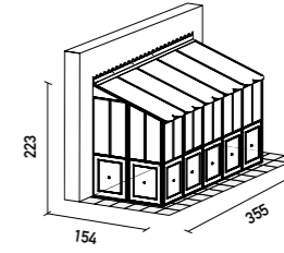
W 355 D 154 H 223
